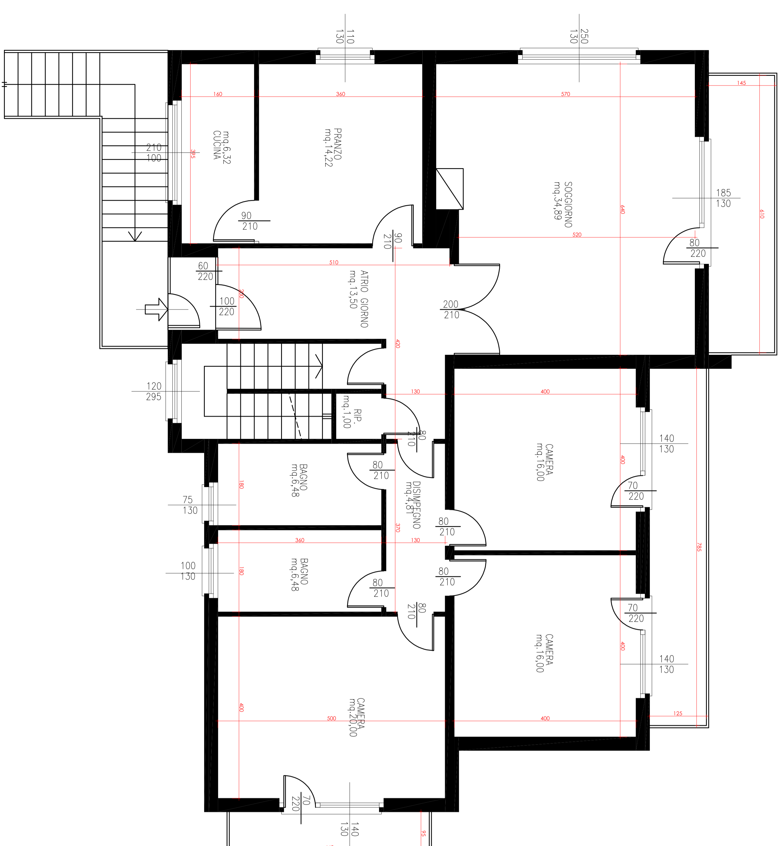
Pianta Piano Primo- Attuale
