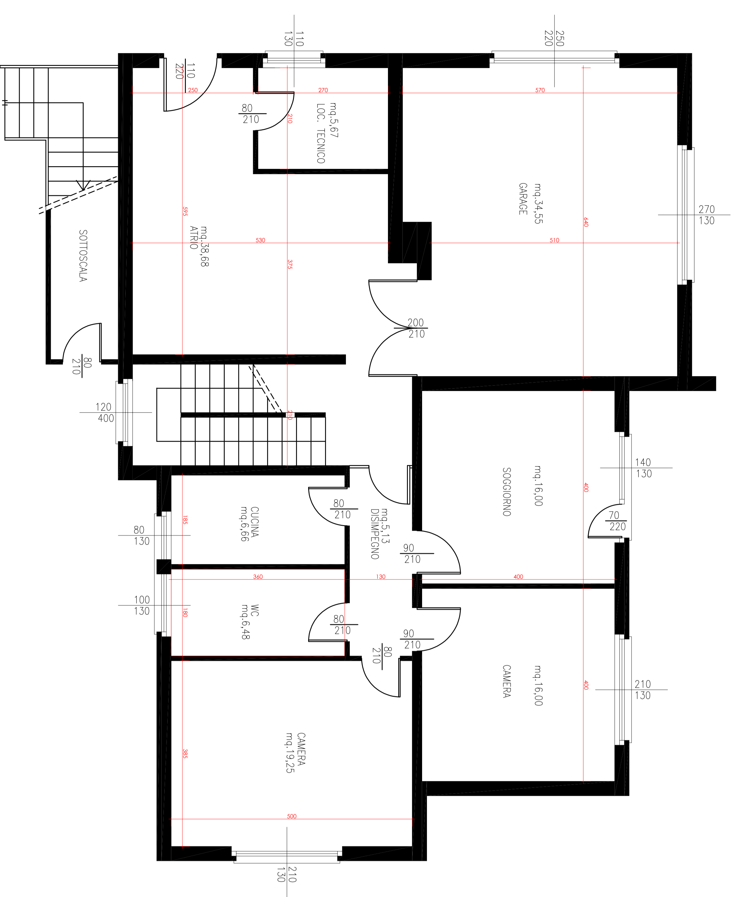
Pianta Piano Terra- Stato Attuale
