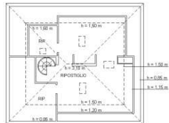
PIANO PRIMO (sottotetto)
